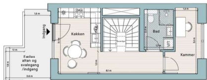
3. sal
