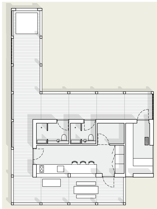
Plan 1 : 150
