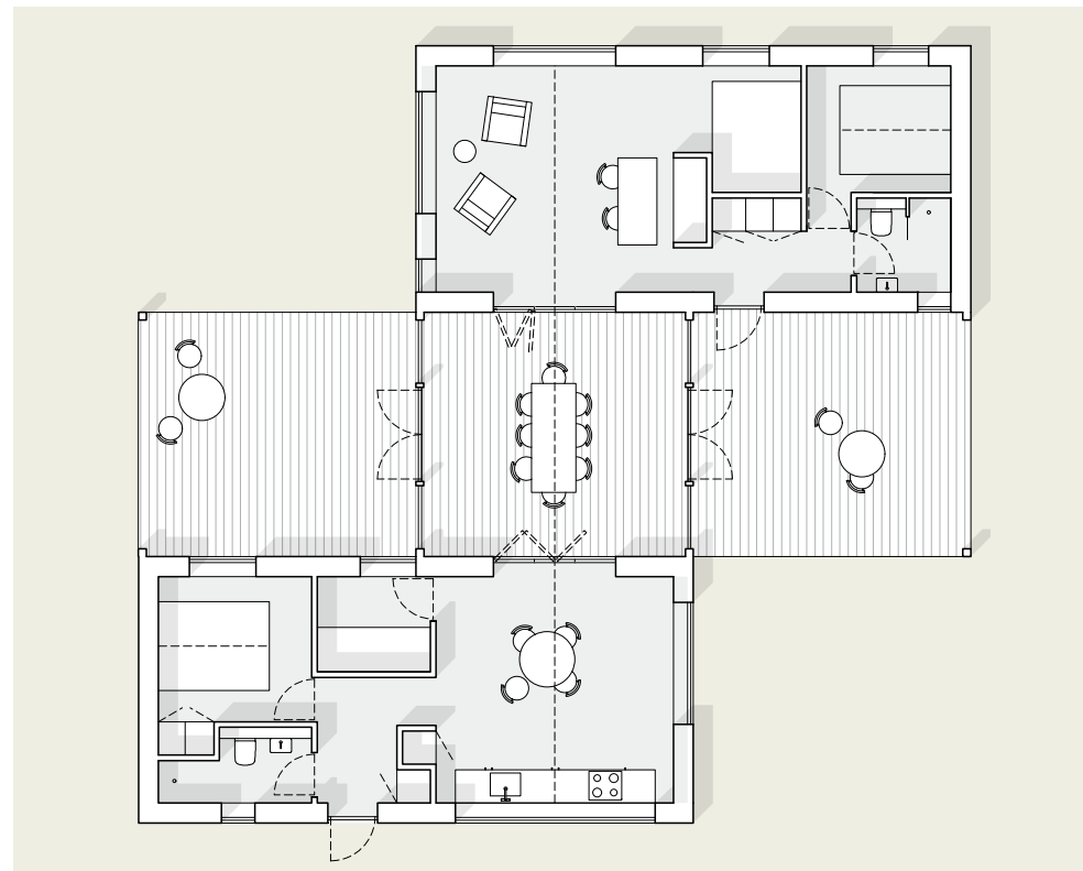
Plan 1:150
