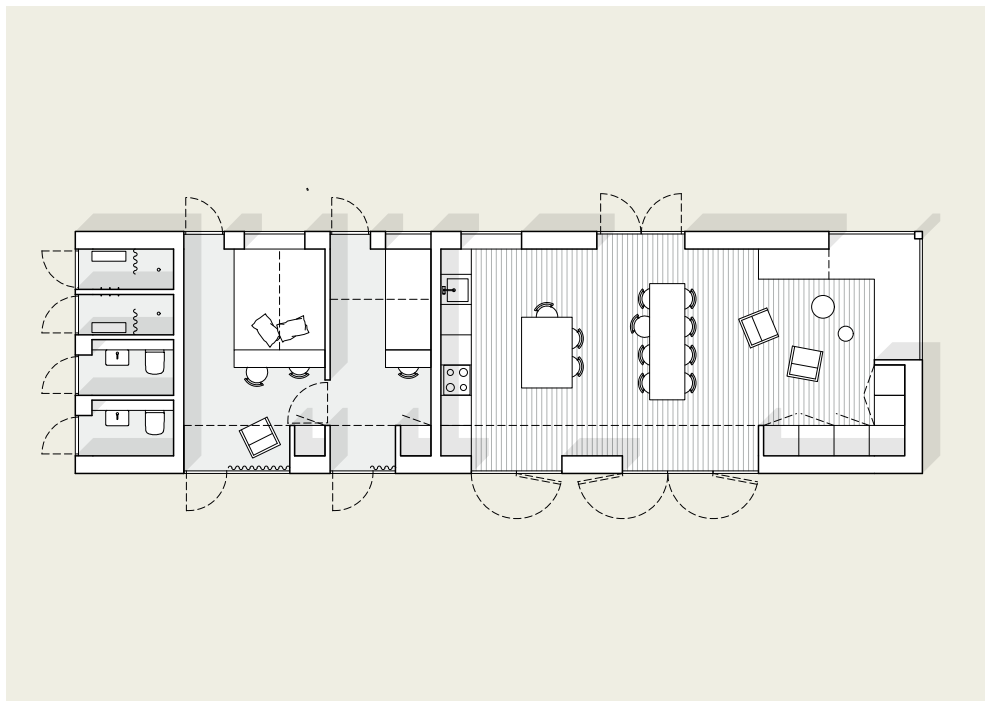
Plan 1:150
